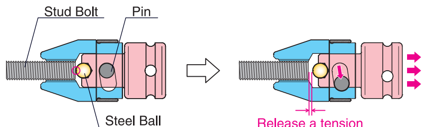
Installing a stud bolt
